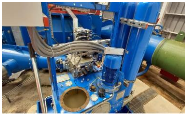
Hidroeléctrica Santa Elena , Villarrica Mantenimiento sistema hidráulico, unidad Pelton. Central Santa Elena
